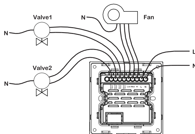
Sơ đồ đấu nối
