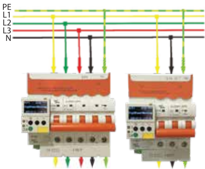
Sơ đồ đấu nối
