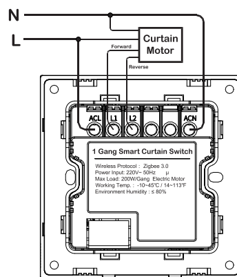
Sơ đồ đấu nối
