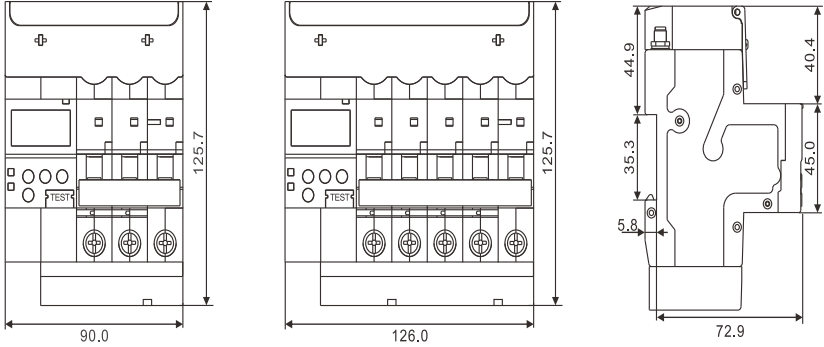
Kích thước sản phẩm (Lắp vừa thanh cài tủ điện)
