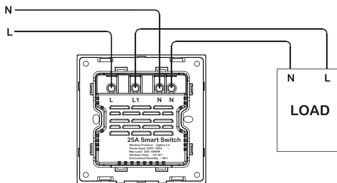
Sơ đồ đấu nối
