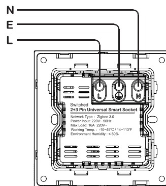
Sơ đồ đấu nối
