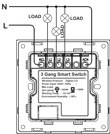
Sơ đồ đấu nối
