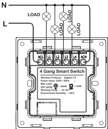
Sơ đồ đấu nối
