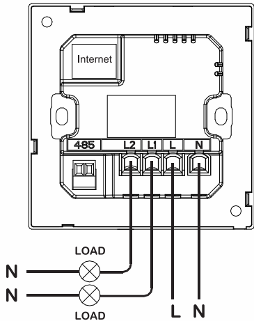
Sơ đồ đấu nối
