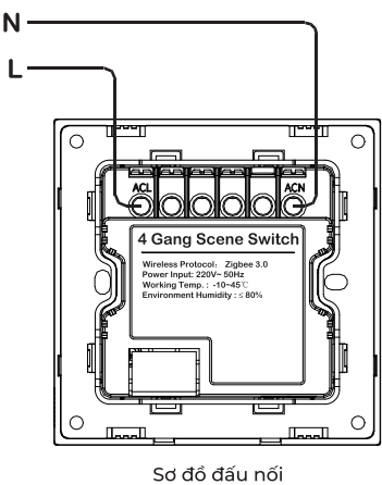
Sơ đồ đấu nối
