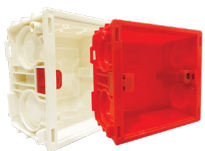
MODEL: 86-P15 16.500 VND Đế âm vuông 86mm KT: 84x86x49mm Có thể lắp ghép dài vô tận Switch & socket wall base box 86mm
